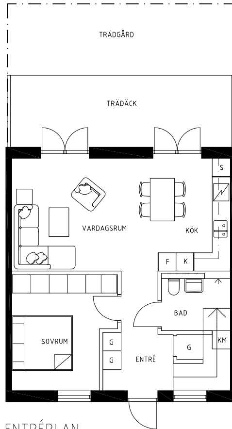
ENTRÉPLAN
