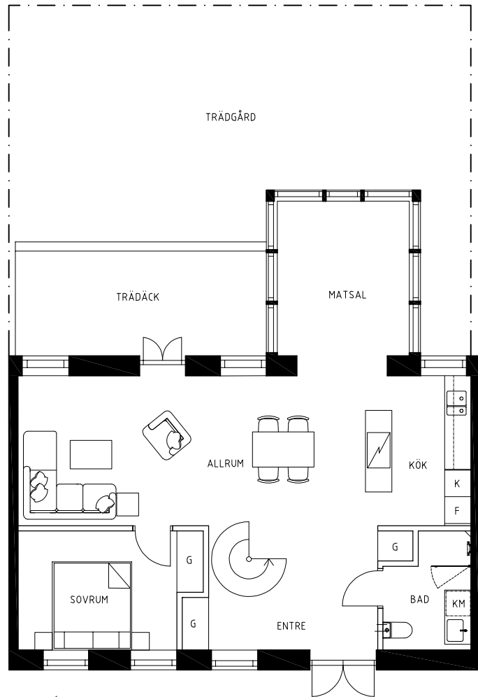
ENTRÉPLAN
