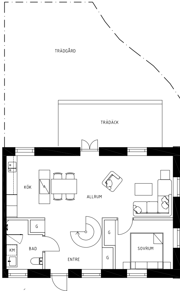
ENTRÉPLAN
