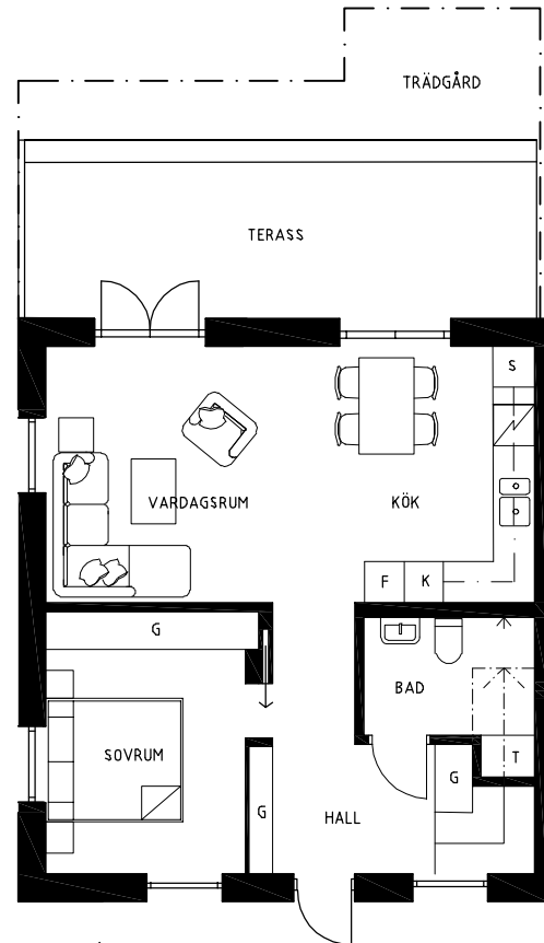
ENTRÉPLAN
